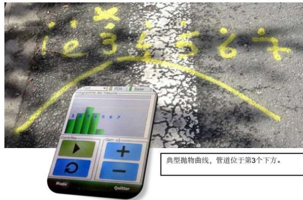
图 4-5 通常情况现场分析图
