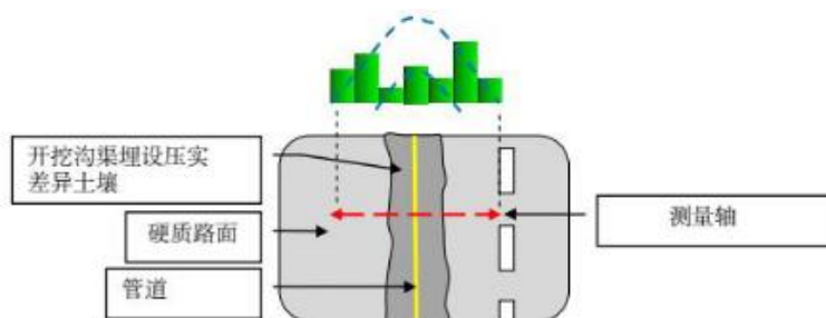
压实区信号示意图
