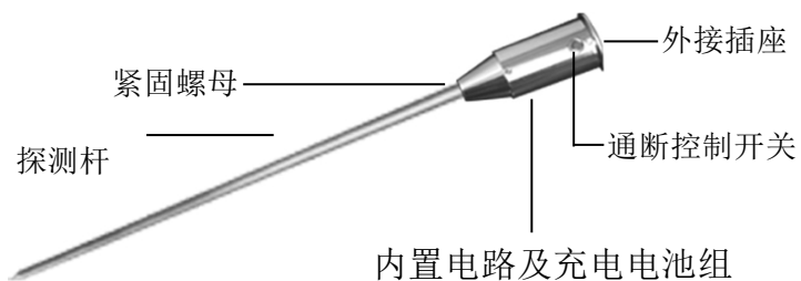
JT-TLD 型听漏棒构成图
