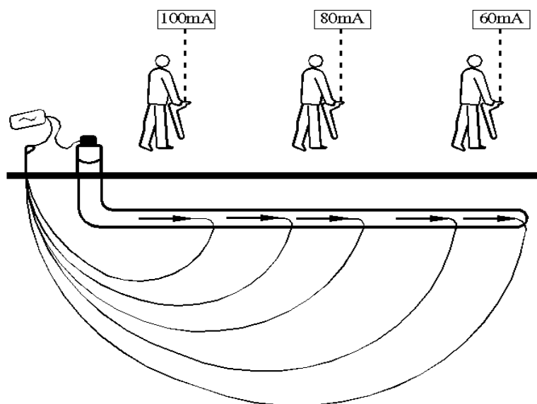
图 h 电流测量原理示意图
